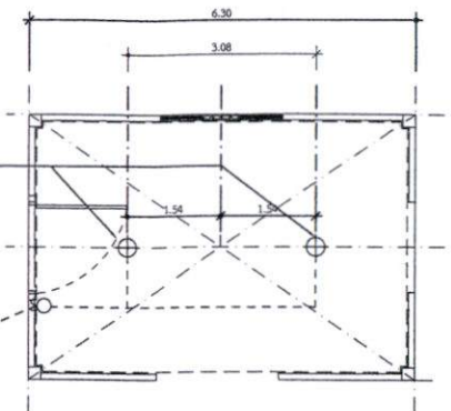
แปลนแปลนไฟฟ้า R มาตราส่วน 1:100
