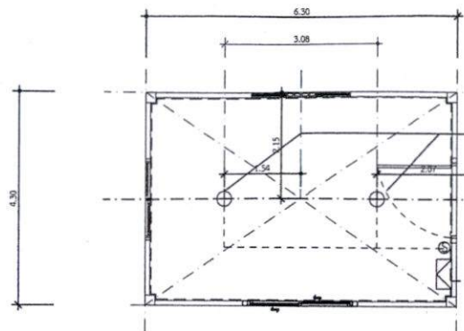
แปลนแปลนไฟฟ้า L มาตราส่วน 1:100
