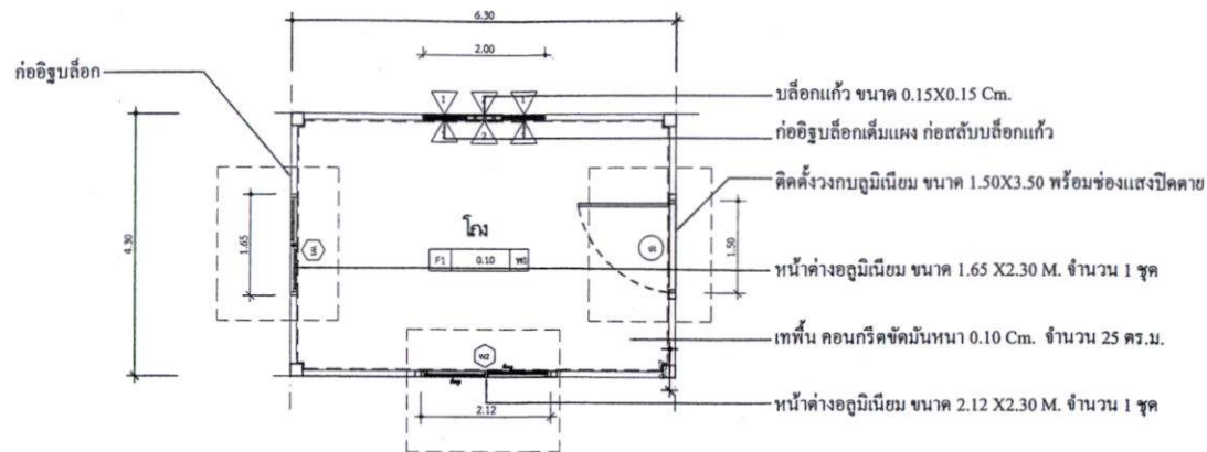
แปลนพื้น 1 มาตราส่วน 1:100
